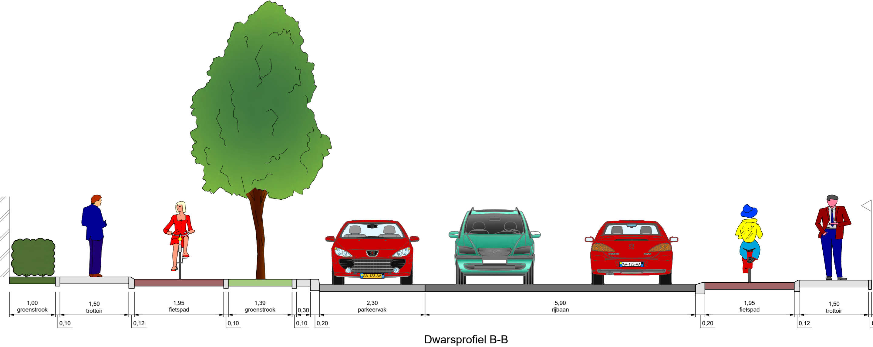
Dwarsprofiel B-B schaal 1:50
