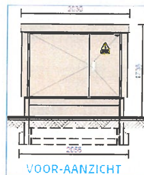
Aanzicht trafo zijde Prealle
