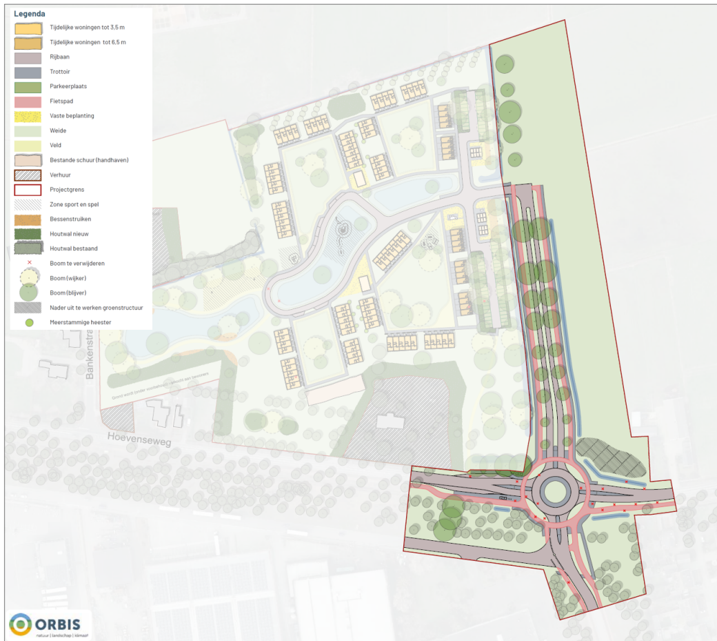
Figuur 2.4 Definitief ontwerp rotonde en ontsluiting.
